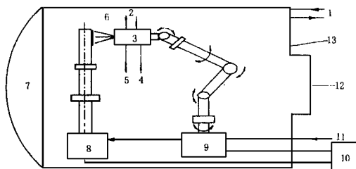
图1 真空室系统示意图
