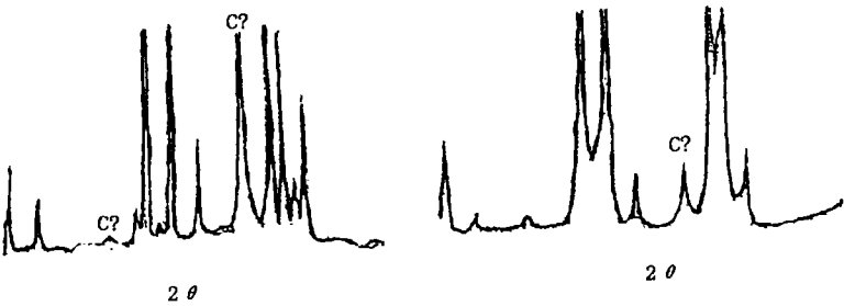
图 2 X 射线衍射图
